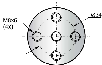
PNB-100-063 - Base de Interligação
